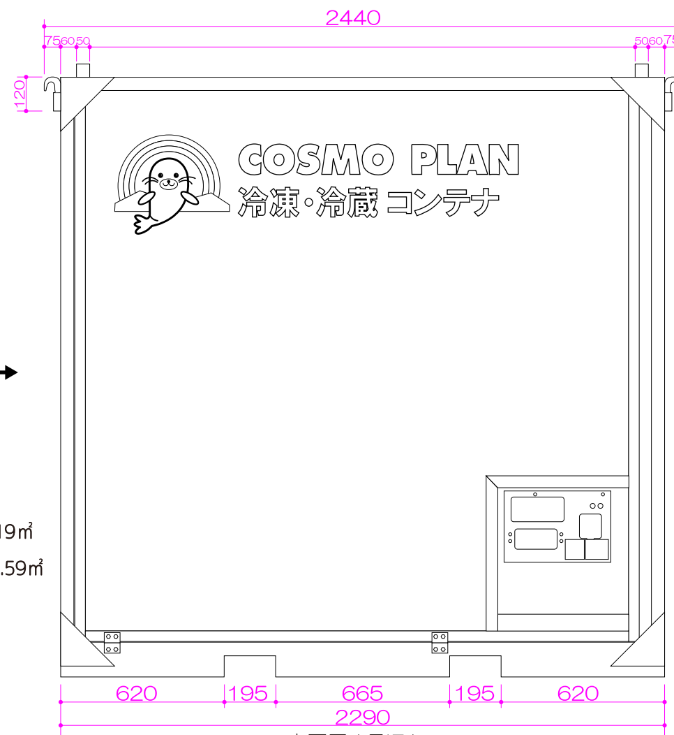
- 立面図 (長辺) -
