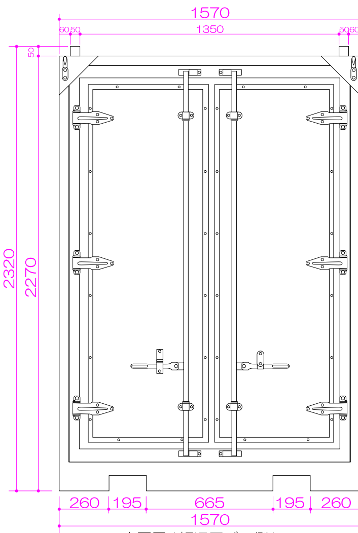
- 立面図 (短辺戸びら側) -
