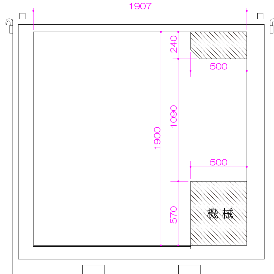
- 断面図 (長辺) -
